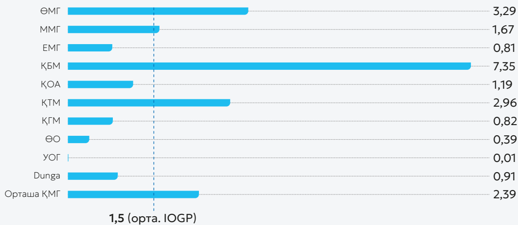
Өндірілетін 1 тонна КСШ-ға энергияның үлестік тұтынуы, ГДж/т
